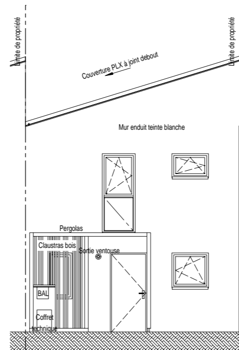
Elévation Est
