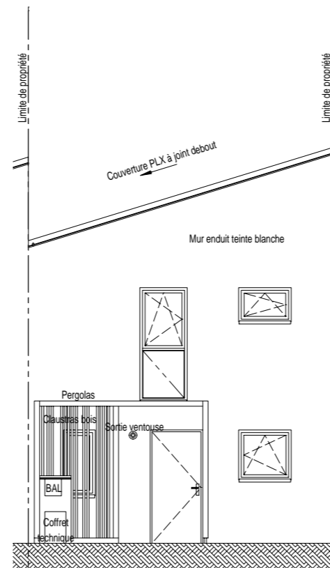
Elévation Est
