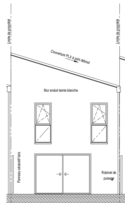
Elévation Ouest
