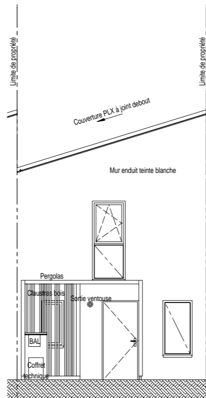
Elévation Est
