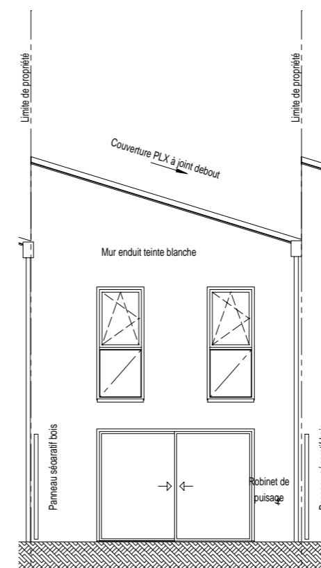
Elévation Ouest
