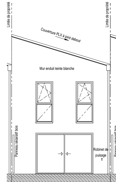
Elévation Ouest
