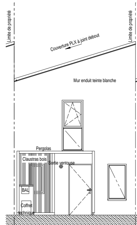
Elévation Est
